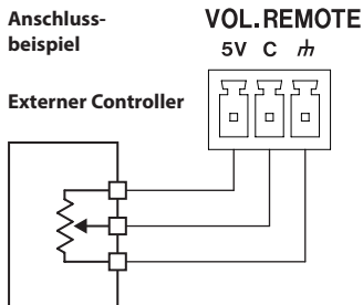
Lautstärke-Potentiometer 10 k \Omega logarithmisch
