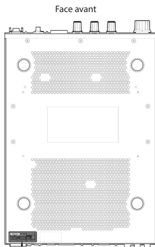
Plaque signalétique
